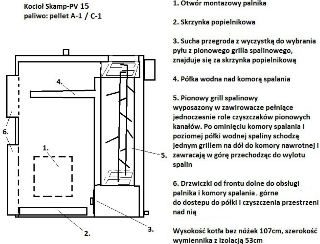
Rys.1. Kocioł "SKAMP-PV"
